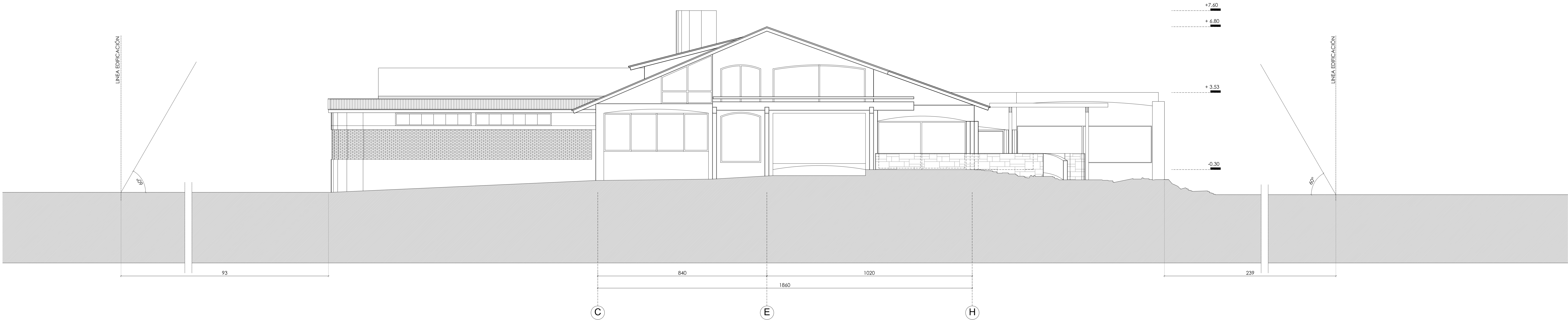
1 ELEVACION PONIENTE
