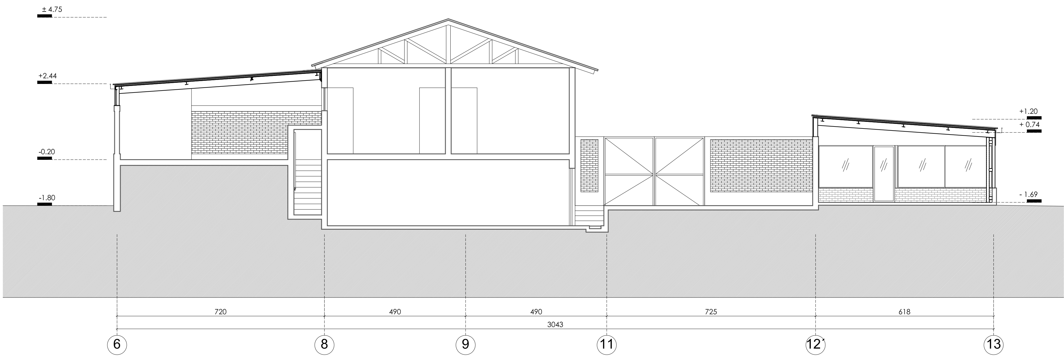
2 CORTE B - B
