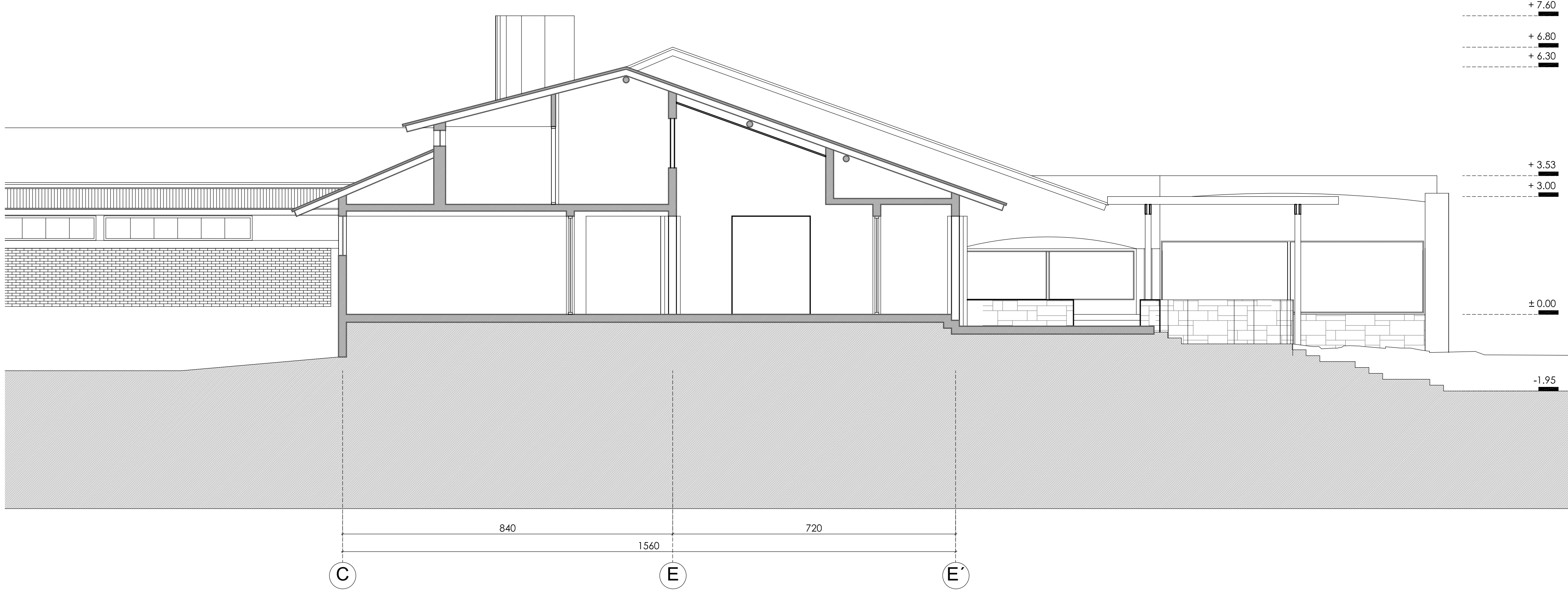
1 CORTE A - A
